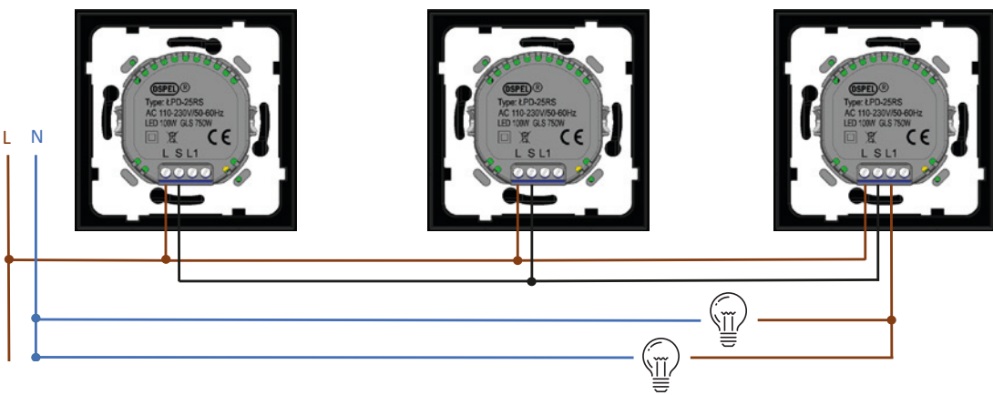
Łączniki dotykowe schodowe funkcja łącznika podwójnego krzyżowego
