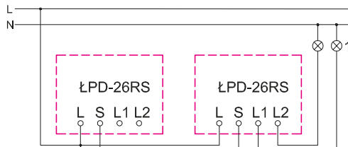
Łączniki schodowe podwójne
