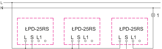
Łączniki schodowe
