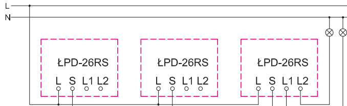
Łączniki schodowe podwójne
