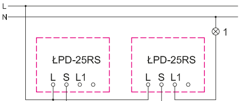
Łączniki schodowe
