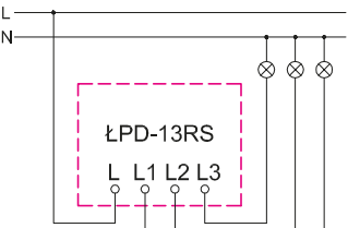
Łącznik potrójny
