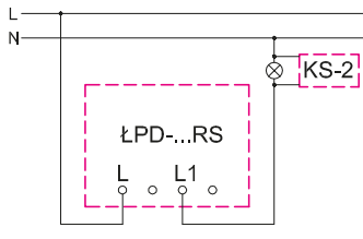
Bypass - przeciwzakłócenia
